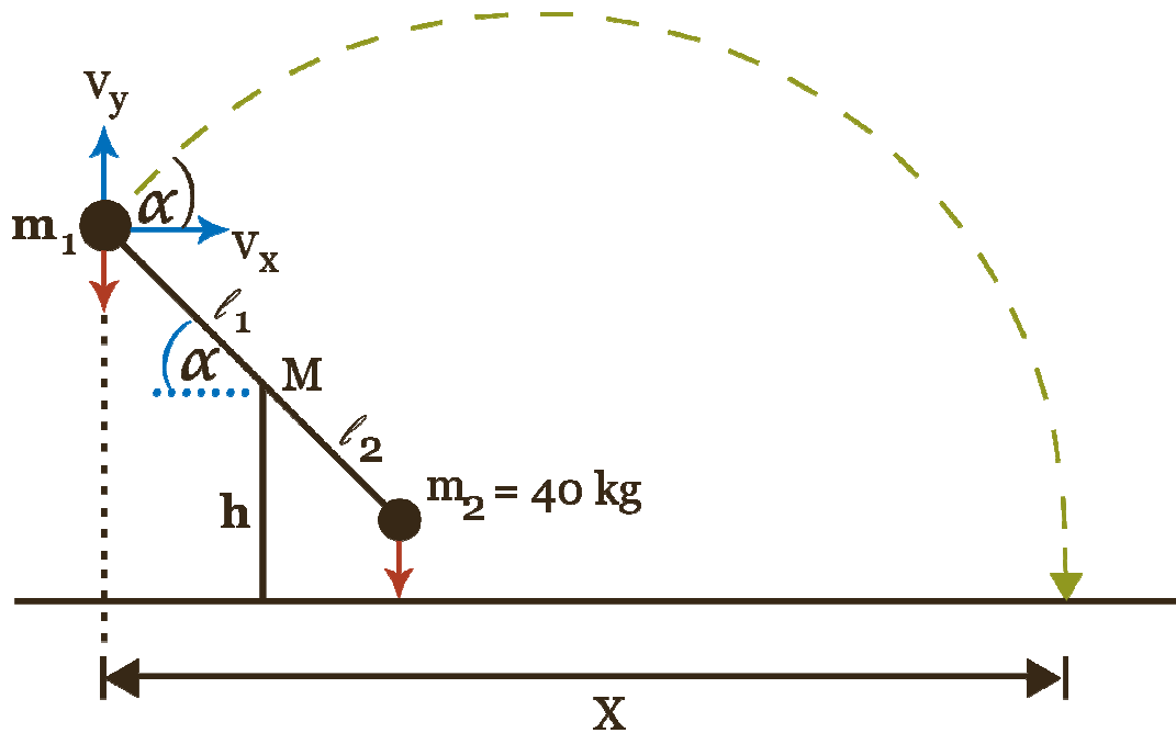
Berechnung der Flugstrecke beim „Fumpinator3000“ mit hier basierenden virtuellen 40kg Gegengewicht. Grafik:by Internet
